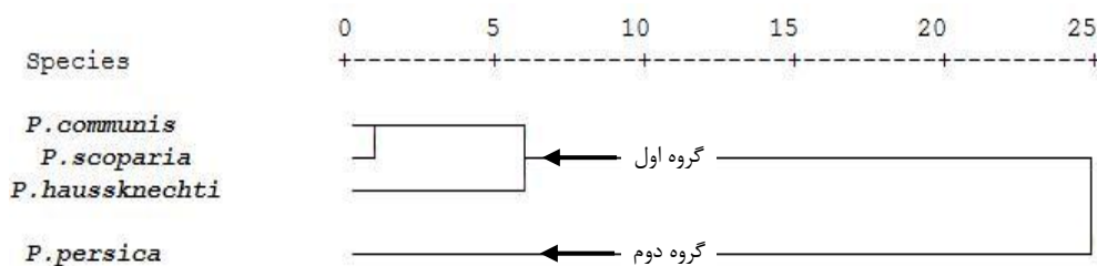
شکل ۵. کلاستر حاصل از مقایسه گونه‌های P. scoparia Spach, P. communis L., P. haussknechtii Bornm و P. persica L. برای تأمین نیاز سرمایی برای جوانه‌زنی با استفاده از فواصل اقلیدوسی و روش Ward.
