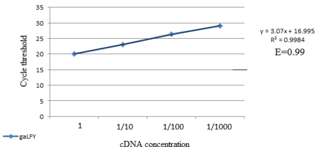
شکل ۳. منحنی استاندارد، شیب‌خط و کارایی جفت آغازگر (E) برای ژن gaLFY Figure 3. Standard curve, slope and primer efficiency (E) for gaLFY
